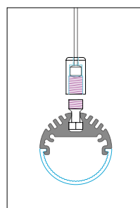
KIT SOSPENSIONE SUSPENSION KIT
