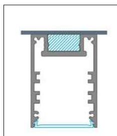
INSTALLAZIONE MAGNETICA MAGNETIC INSTALLATION
