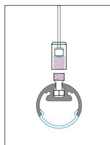
KIT SOSPENSIONE CON SET COPRICAPO SUSPENSION KIT WITH COVER SET
