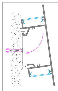
MONTAGGIO A PARETE SU BASETTA WALL-MOUNTED ON PLATE
