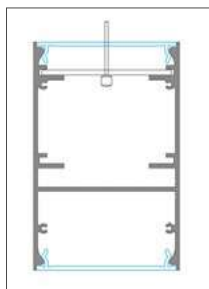
MONTAGGIO A SOSPENSIONE SUSPENDED
