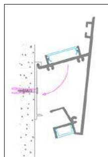
MONTAGGIO A PARETE SU BASETTA WALL-MOUNTED ON PLATE
