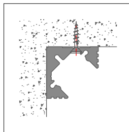
A PARETE CON VITE PROFILE SCREW
