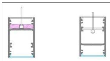
MONTAGGIO A SOSPENSIONE SUSPENDED
