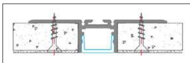
MONTAGGIO AD INCASSO FLUSH-MOUNTED
