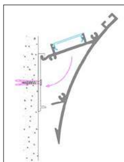
MONTAGGIO A PARETE SU BASETTA WALL-MOUNTED ON PLATE
