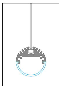
KIT SOSPENSIONE CON SET COPRICAPO SUSPENSION KIT WITH COVER SET
