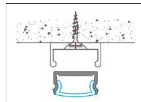
MONTAGGIO AL SOFFITTO CON CLIP CEILING-MOUNTING WITH CLIPS
