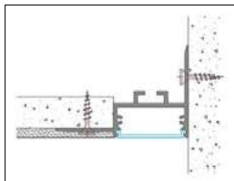
MONTAGGIO A PARETE / CARTONGESSO RECESSED
