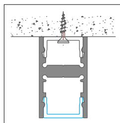
MONTAGGIO AL SOFFITTO CEILING-MOUNTING
