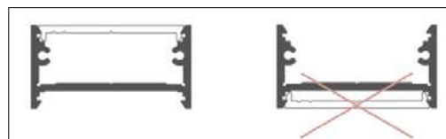
NP024 (NON È POSSIBILE INSTALLARE LA COPERTURA SUL LATO STRETTO) NP024 (COVER CANNOT BE INSTALLED ON NARROW SIDE)
